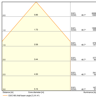
PL FLEX 600 S 17W 3000K U19 2830lm
